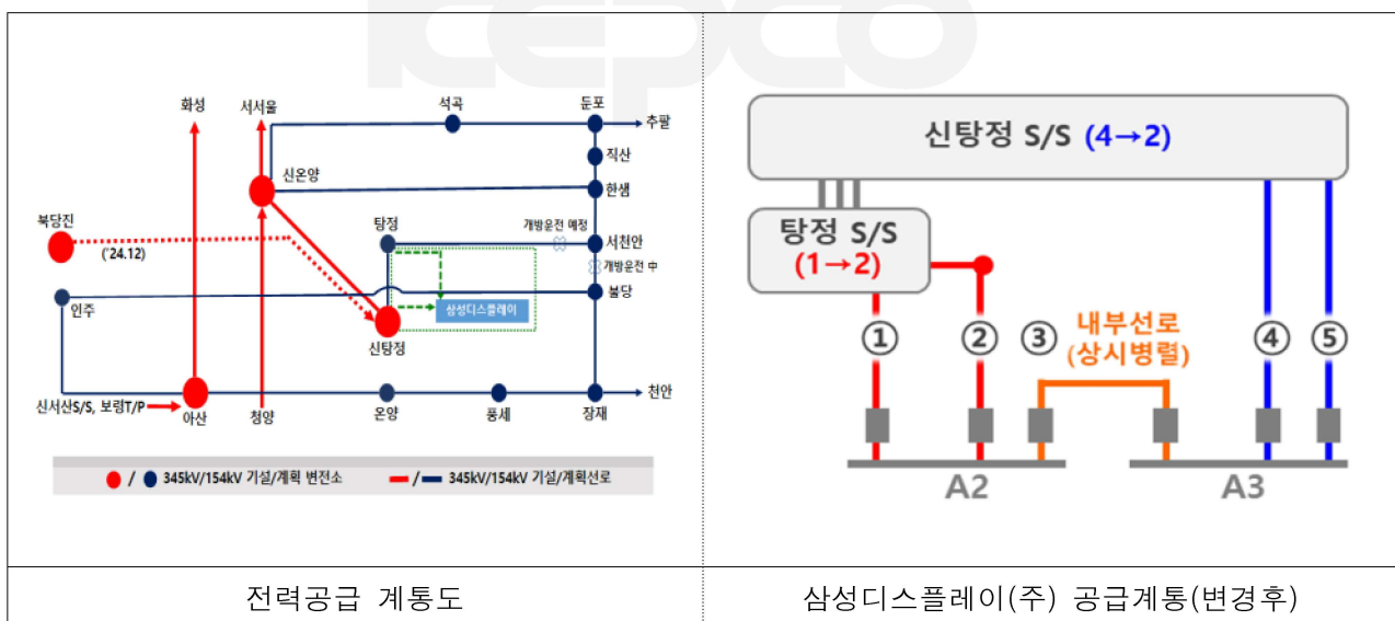
[그림2] 삼성디스플레이(주) 전력계통 구성(後)
